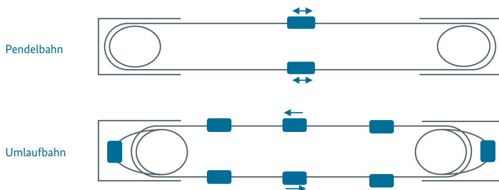
Abbildung 10: Funktionsprinzip Seilschwebebahnen
