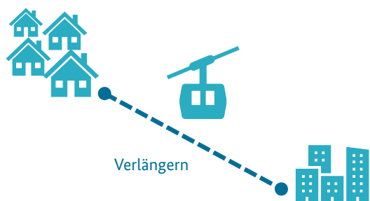
Abbildung 4: Anwendungsfall „Verlängern“
